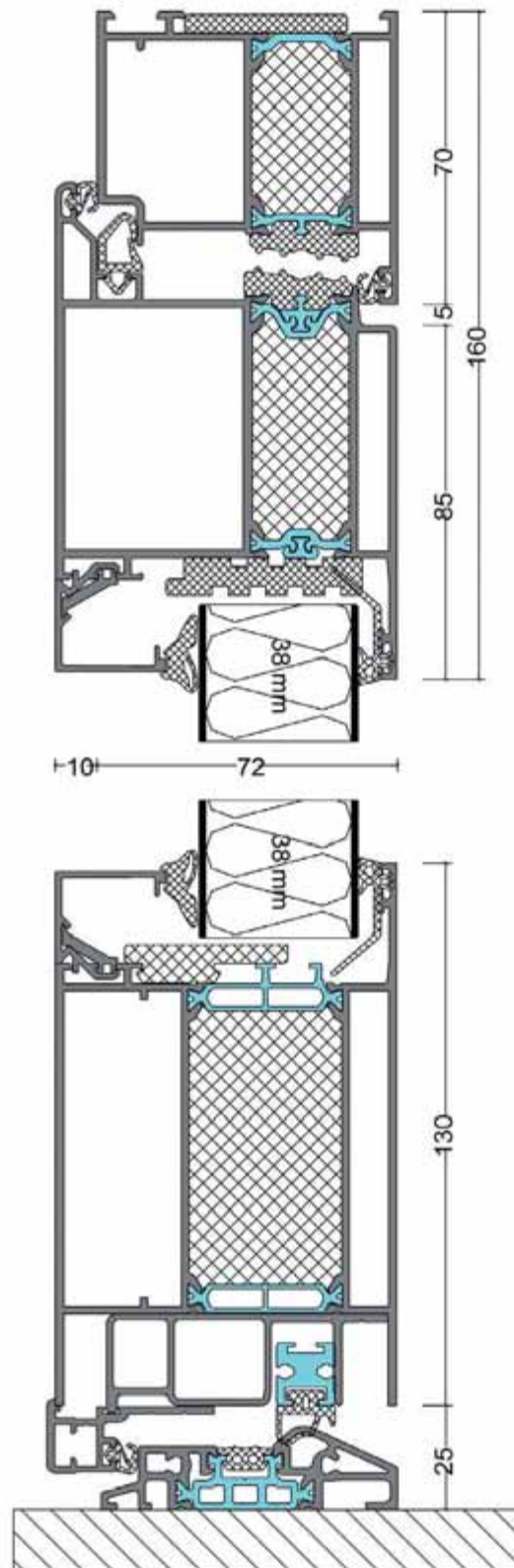
Außenansicht Blendrahmen gerade Türflügel gerade
