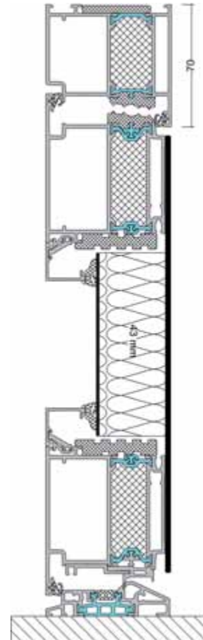
Außenansicht Blendrahmen gerade Türflügel außen überdeckt
